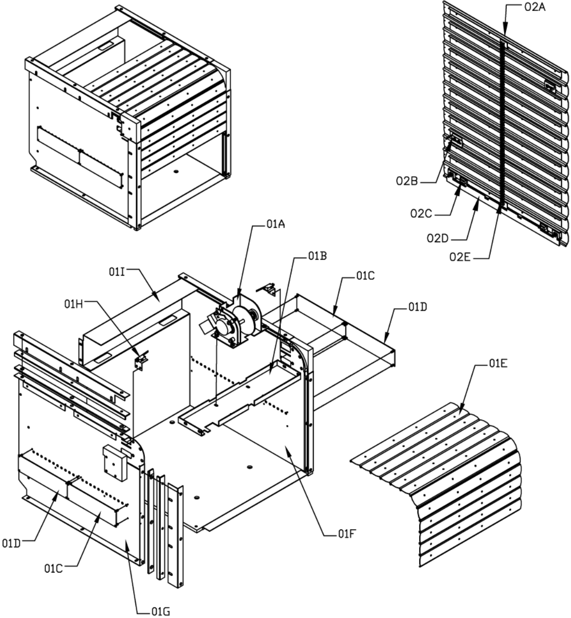
01. ROLLING DOOR ASSEMBLY
