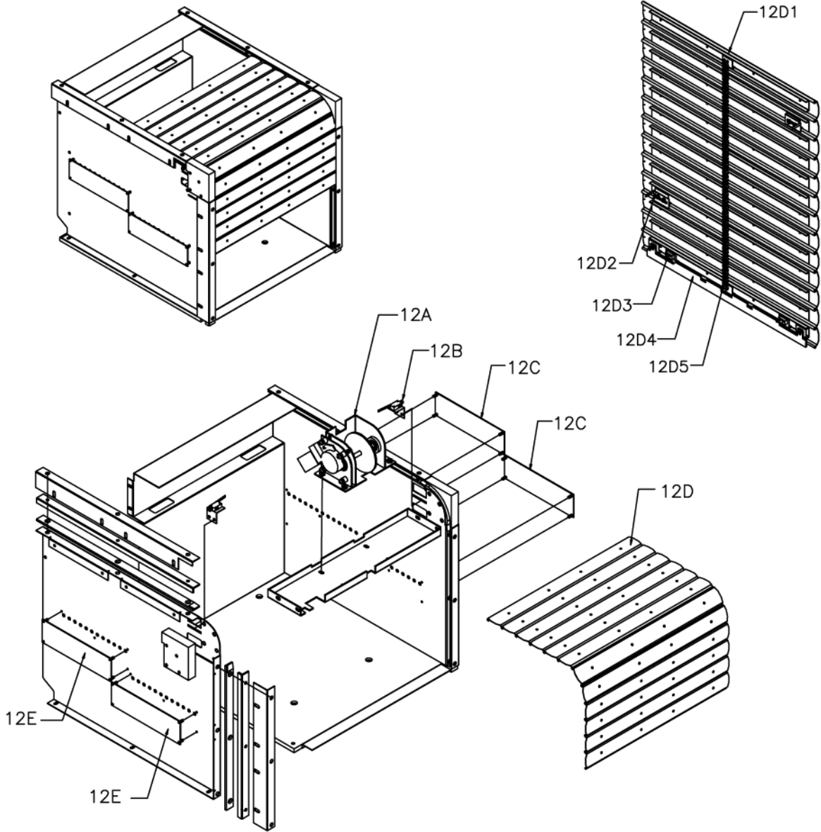
12. LHG A006 ROLLING DOOR ASSEMBLY
